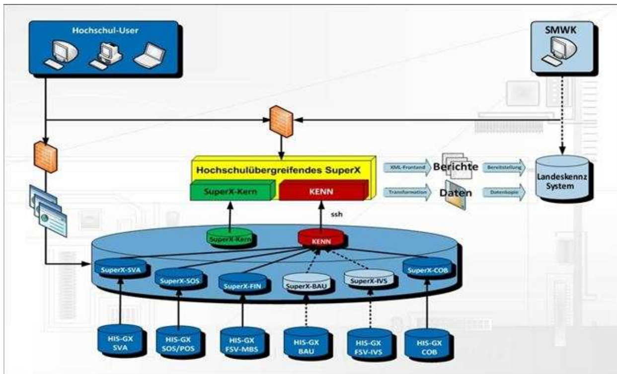
Abb. 5 Architektur für hochschulübergreifende SuperX-Instanz
