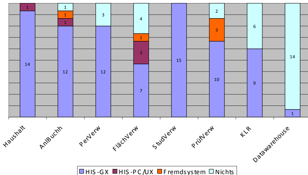
Abb. 1 Software-Profil
